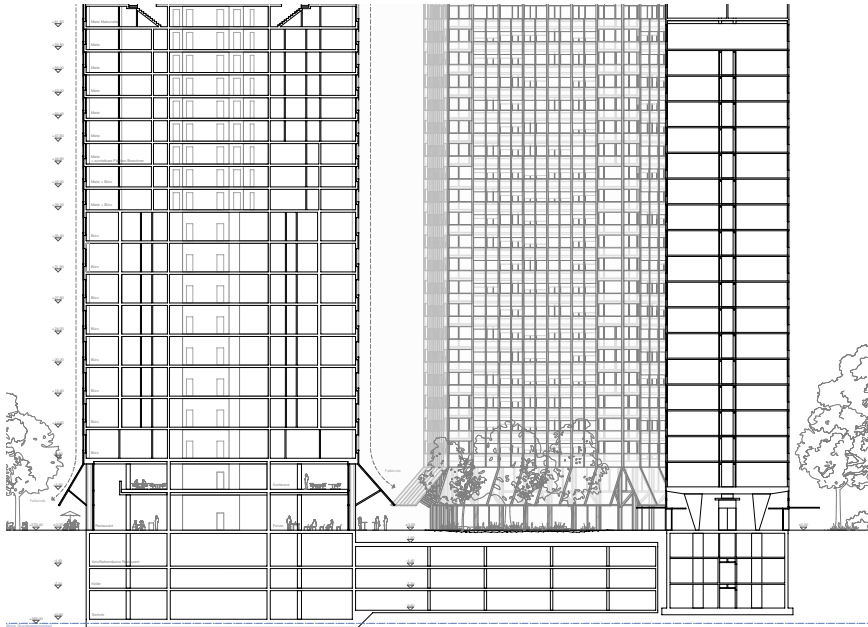
Querschnitt Baufelder C + A
