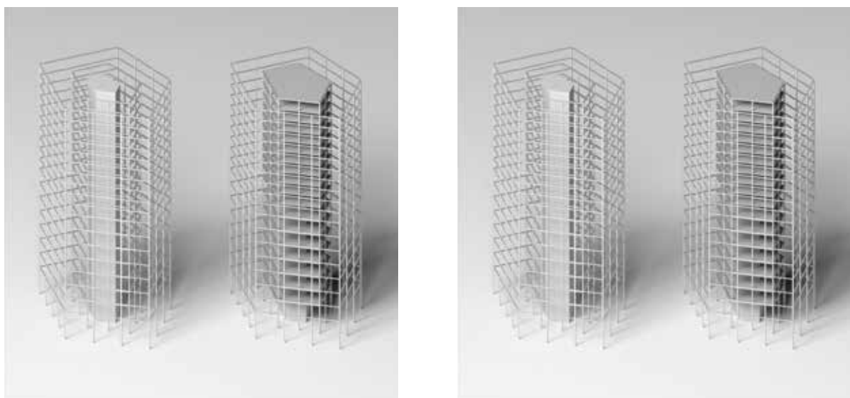
Tragwerkskonzept
