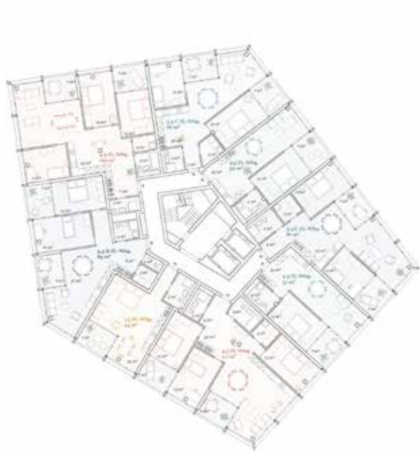
Grundriss Wohnen Baufeld C (7.-17. OG)
