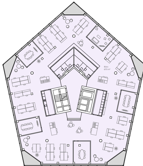
Grundriss Grossraumbüro Baufeld B (5.-9. OG)
