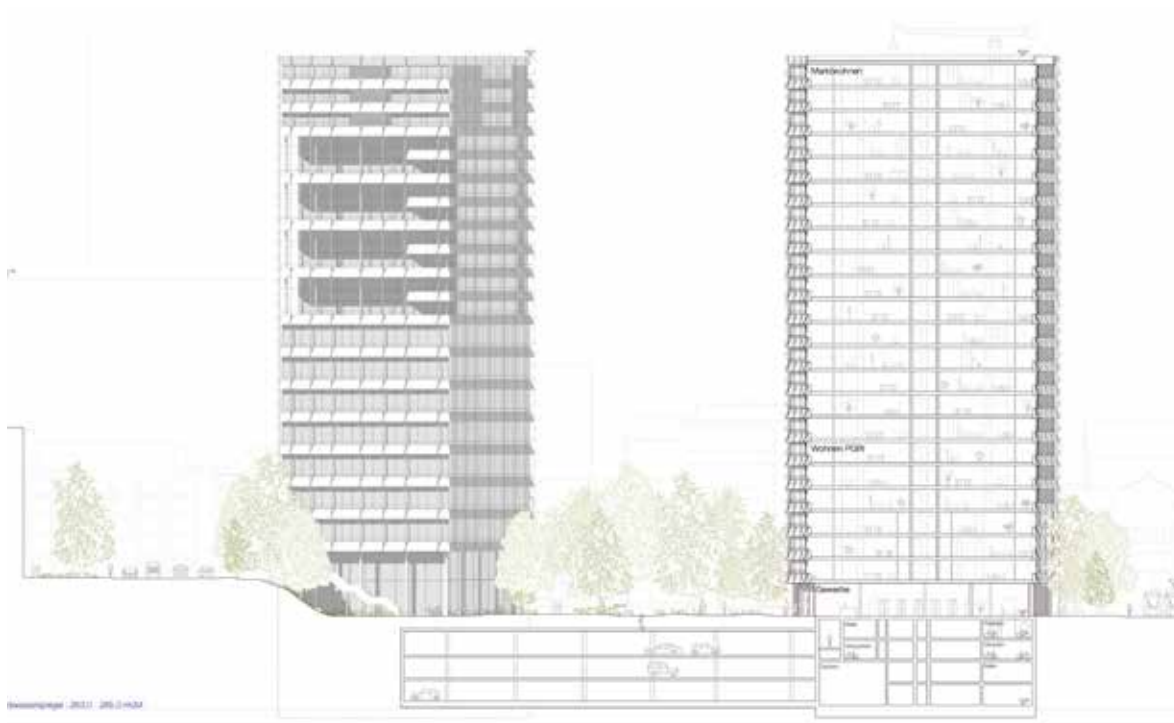
Querschnitt Baufeld C
