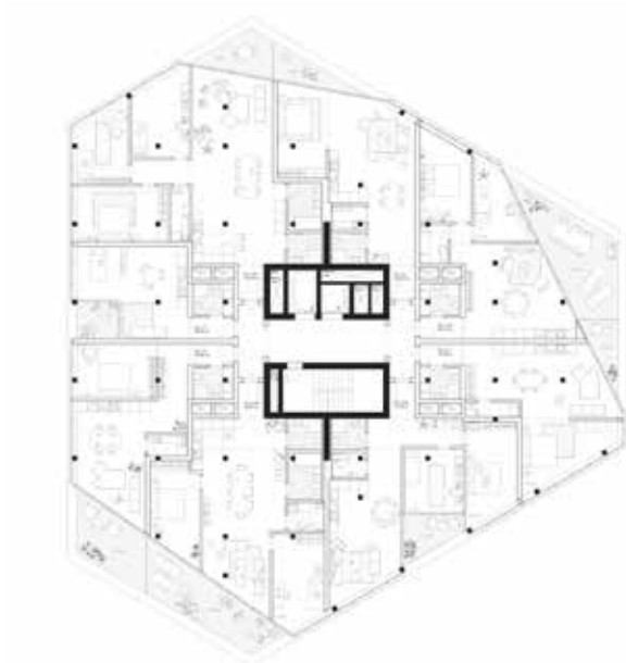
Grundriss Wohnen Baufeld B (14-19. OG)
