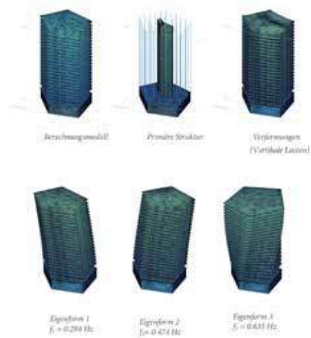
Statisches Modell
