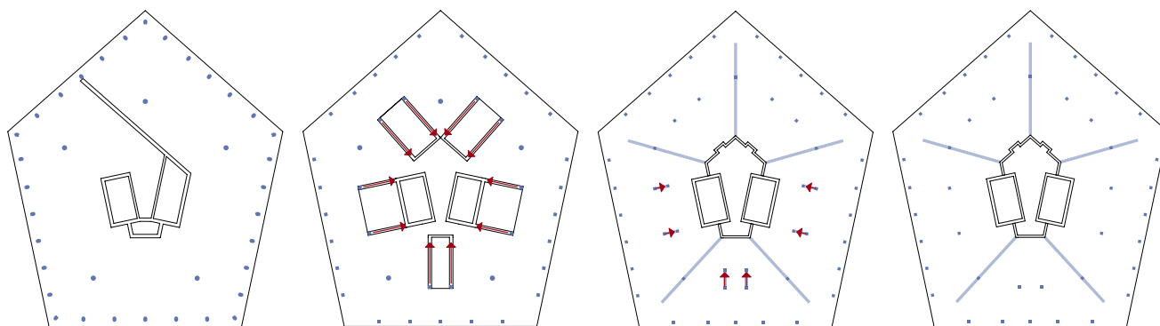
Tragwerkskonzept
