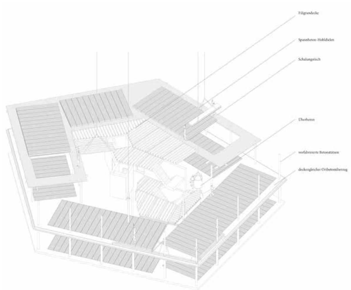
Konstruktion und Bauablauf
