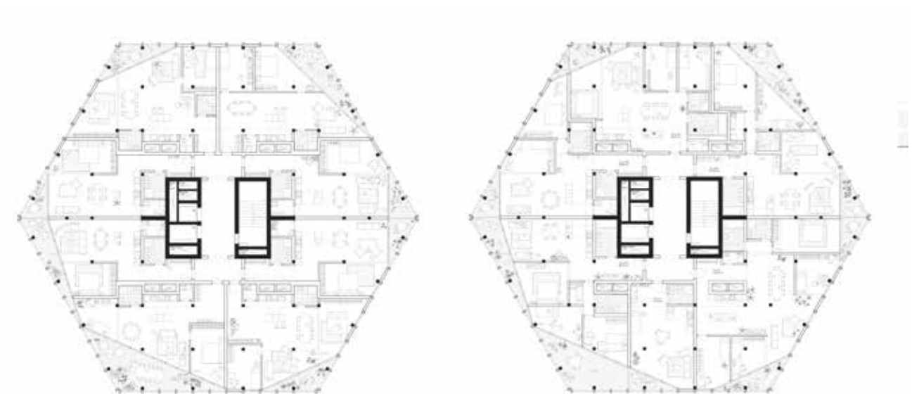
Grundriss Wohnen Baufeld C (15-22. OG)
